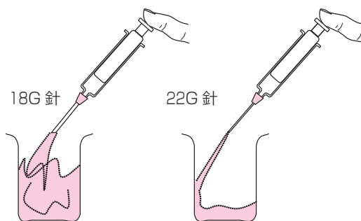
注射針の太さの変化による流量変化 『最新臨床工学講座 医用機械工学』より
