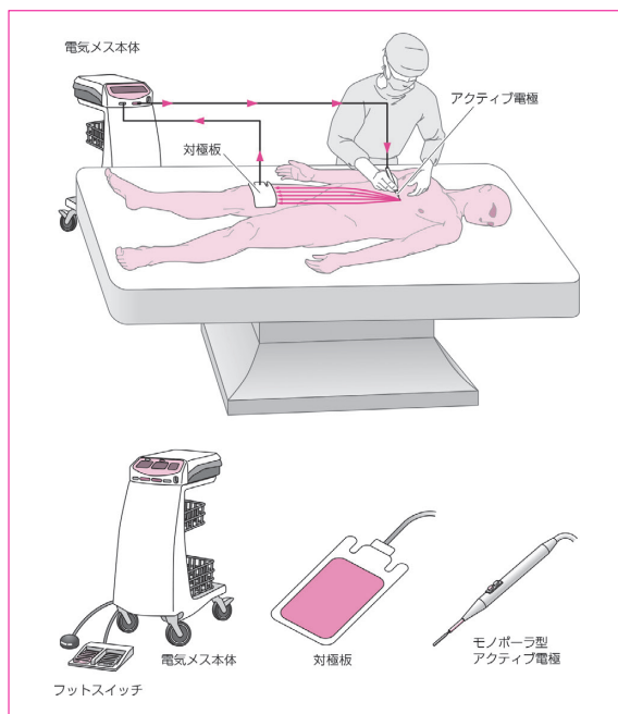
電気メスの構成 『最新臨床工学講座 医用治療機器学』より
