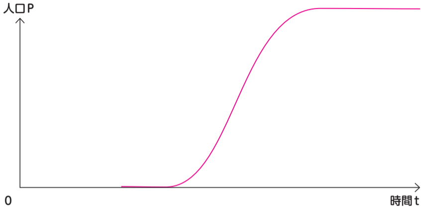
図9-3 フェルフルストの人口モデル（ロジスティック方程式）に従った人口推移
